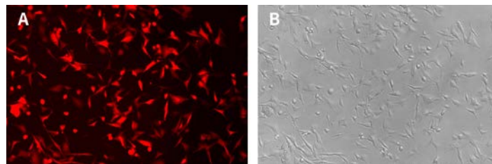
图1. 碧云天STAT3-TA-Luc-EF1 \alpha -mCherry U-87 MG Cells (C8305) 的荧光显微镜观察图。A为荧光照片, B为明场照片。实际检测效果会因检测仪器、实验条件的不同而存在差异, 本图仅供参考。
